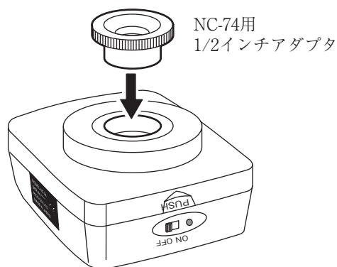
音響校正器 NC-74
